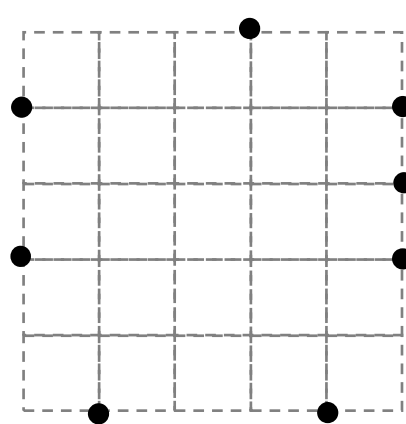
二等辺三角形
