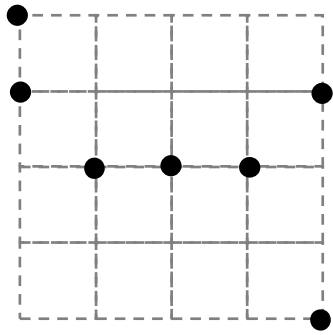
二等辺三角形
