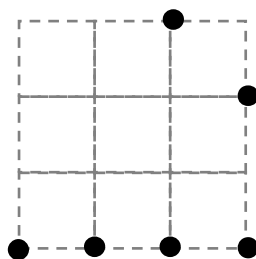
直角二等辺三角形
