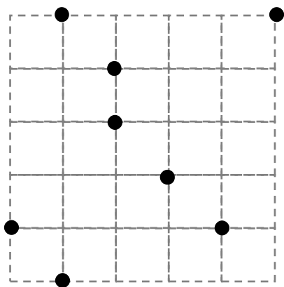
直角二等辺三角形
