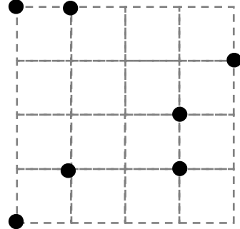
二等辺三角形
