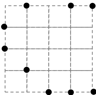
直角二等辺三角形
